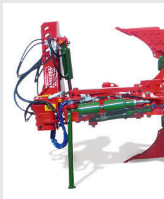
Ajuste 1º surco hidráulico especial para pendientes (*).
